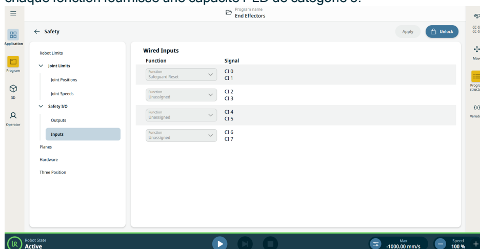
Figure 1.4: Écran PolyScope X affichant les signaux d'entrée.
