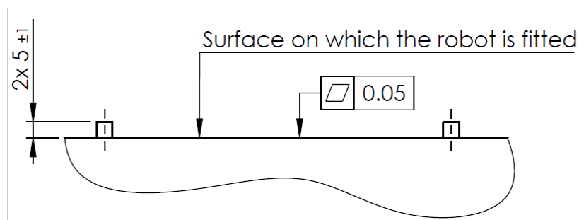
1.2: Plaque de montage pour base de robot
