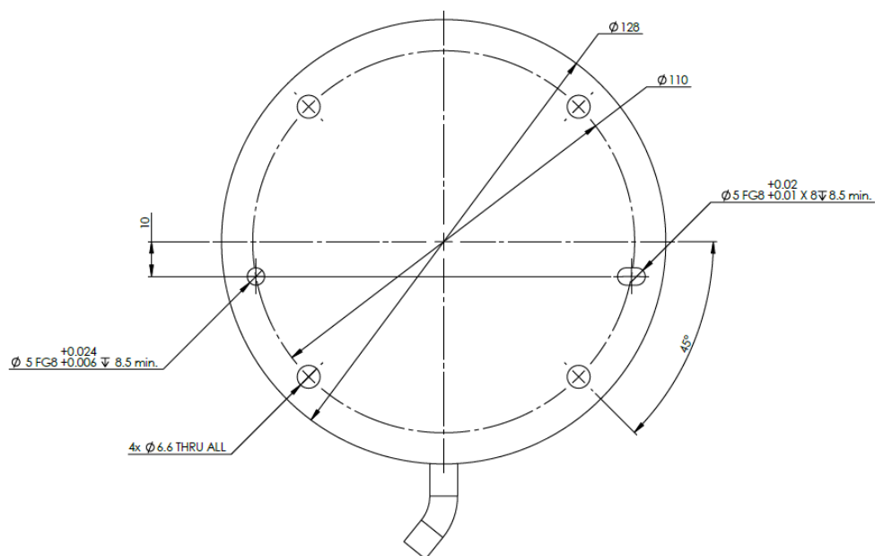
1.1: Vue de dessous de la base du robot
